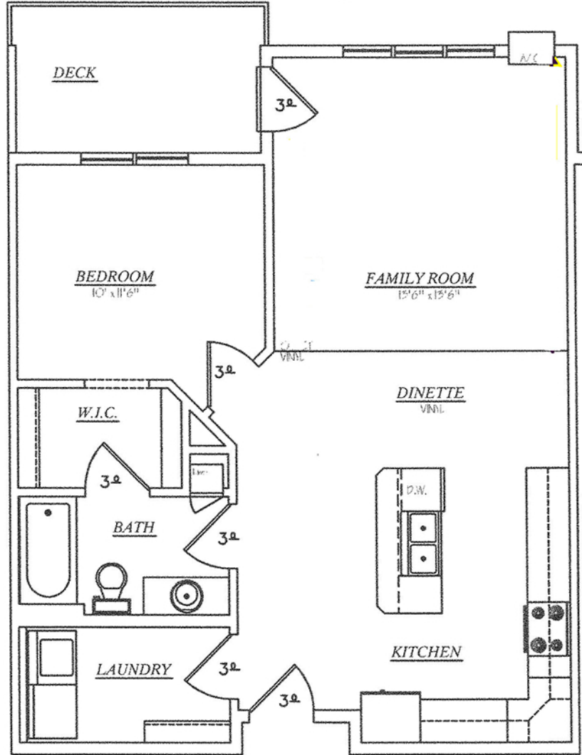
1-BEDROOM - UNIT A SCALE: 1/8" = 1'-0" 810 SQFT
